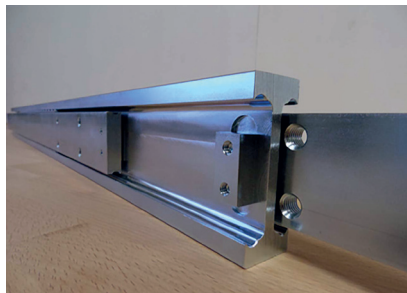
Teleskopschienen der 4Linear GmbH
