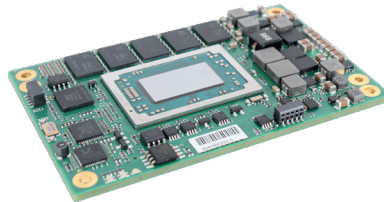
Emerson mini COM Express Module - mCOM10-L1900 (AMD V1000)
