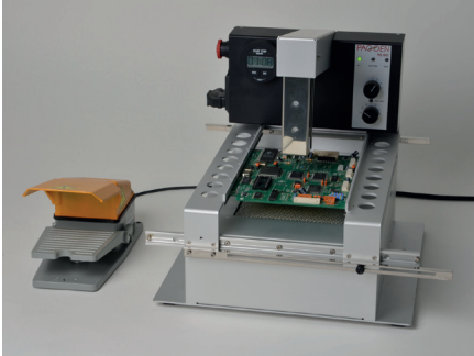
Reparatur- und Rework System
